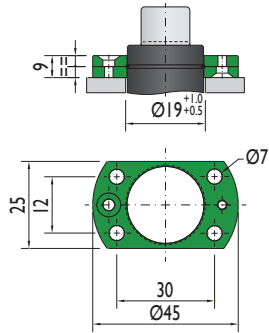
XQ-100
