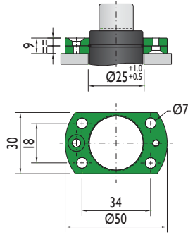
XQ-200
